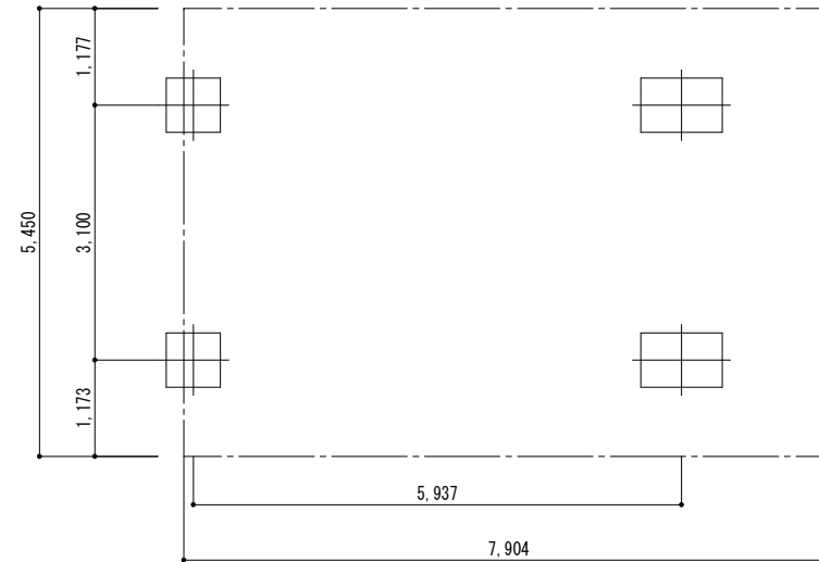
■基礎配置図
